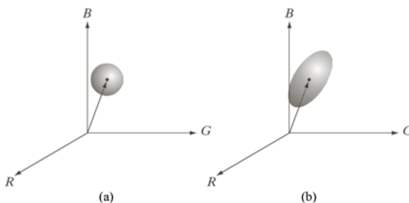
Slika 18: Evklidska in Mahalanobisova razdalja (Gonzales in sod., 2004).
