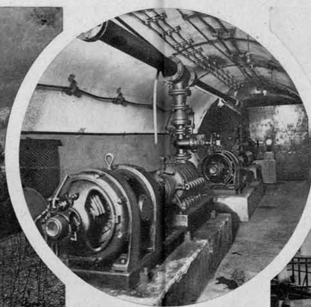
Rudniške sesalje za vodo v Trbovljah.
