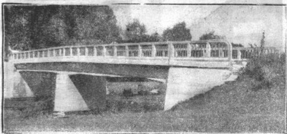
Lansko leto zgrajeni železobetonski most čez Poljansčico v Škofji Loki, ki ga je povodenj podrla in gornji del odnesla 40 m daleč po vodi, kjer se je zaril v zemljo, a se ni razbil.
