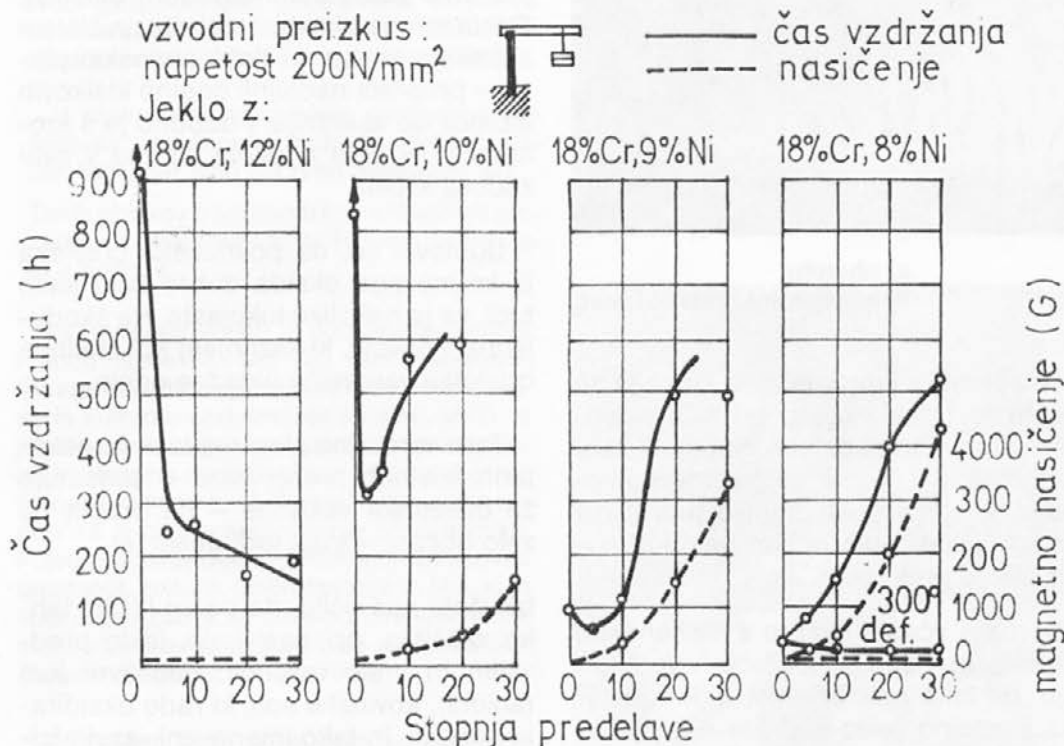
Sl. 3 Hladna predelava pusti v jeklu napetosti, ki zmanjšujejo obstojnost proti zunanji napetosti in koroziji (leva slika). Če nastaja med hladno deformacijo martenzit, zboljšuje s svojim potencialom nasproti avstenitu obstojnost proti napetostni koroziji. Preizkušali so v vroči vodni raztopini 60 % CaCl + 0,1 % HgCl.
