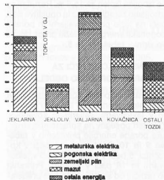
Sl. 5: Struktura porabe energije v letu 1988 za posamezne proizvodne enote
