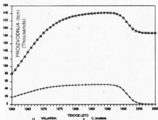
Sl. 3: Sprememba asortimenta jekla v valjarni
