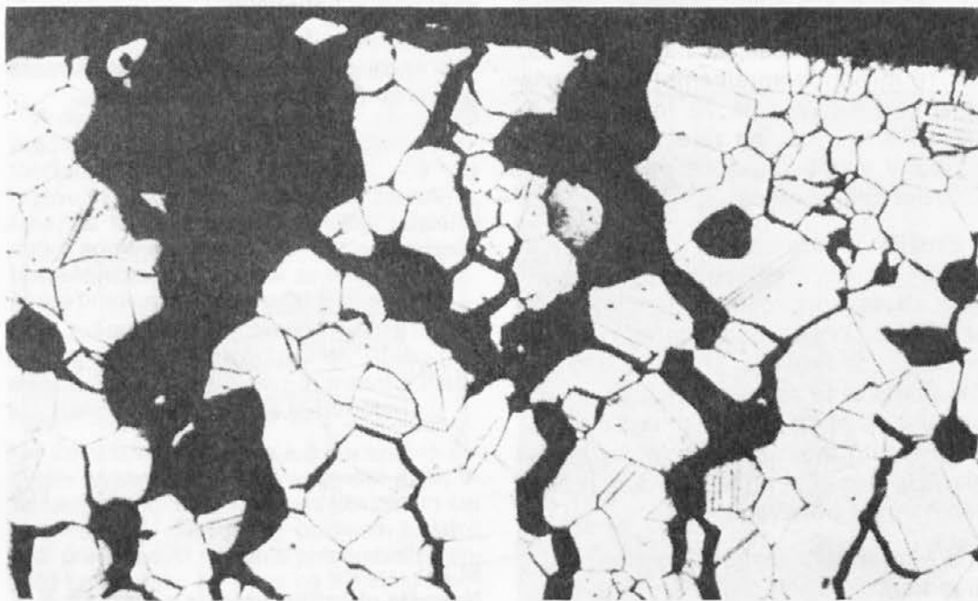
Sl. 4 Mikrostruktura izdelka, ki je poškodovan z medzrnasto korozijo. Glavni notranji vzrok za to korozijo je določena količina ogljika. Nevarno območje, v katerem se tvorijo karbidi, ki ropajo iz zrn kroma, je med 500 in 800°C, bodisi med toplotno obdelavo bodisi varjenjem.
