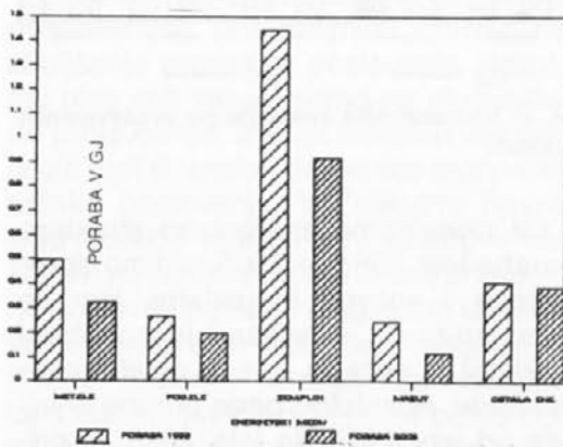
Sl. 9: Sprememba porabe posameznih energetskih medijev
