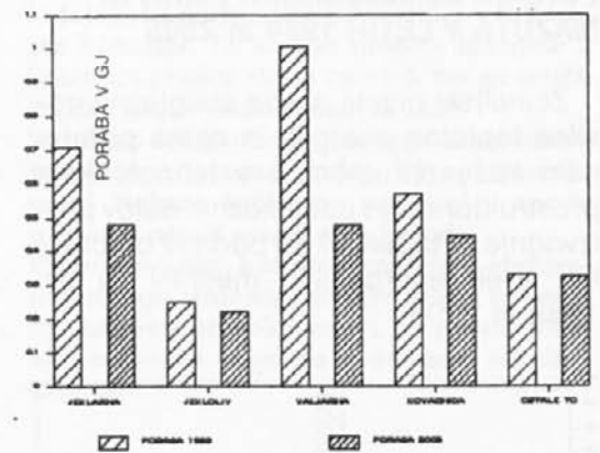
Sl. 7: Sprememba energije po proizvodnih enotah
