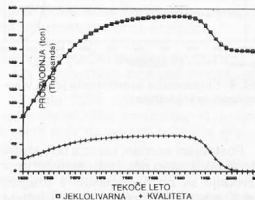
Sl. 2: Sprememba asortimenta jekla v jeklarni
