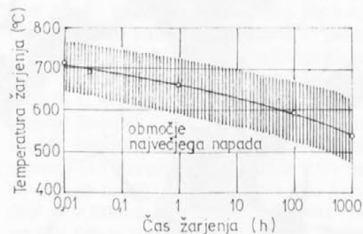
Sl. 6 Največja občutljivost jekla z 18 % Cr, 8 % Ni in zelo malo ogljika proti medzrnasti koroziji je po 500 žarjenja pri 550°C. Odvisnost od časa in temperature je podobna kot pri procesih izločanja novih faz in obstoječih strukturnih delov. To kaže na krivdo izločanja karbidov za razpad zrn.
