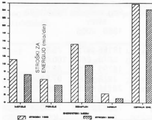
Sl. 11: Razmerje stroškov med posameznimi energetskimi mediji
