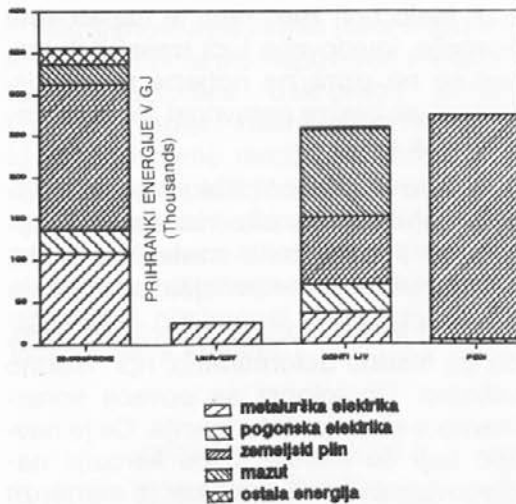
Sl. 14: Prikaz strukture energetskih prihrankov za posamezne investicije in scenarij prihodnjega razvoja železarne
