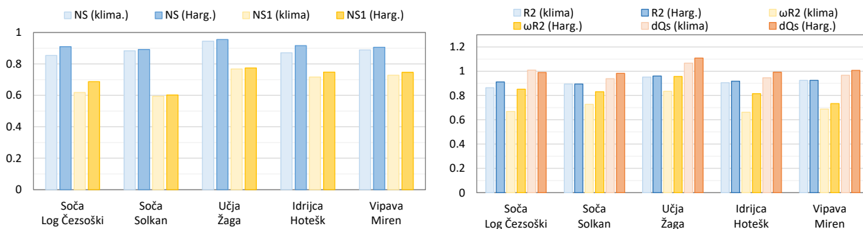
Slika 6: Primerjava uspešnosti simulacij modela Soče ob uporabi dveh različnih virov PET na izbranih vodomernih postajah.
