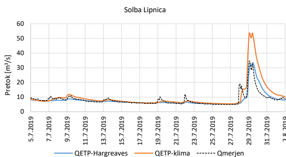
Slika 12: Primerjava simuliranega pretoka z upoštevanjem klimatoloških vrednosti PET in dnevni vrednosti PET z izmerjenimi pretoki na vodomerni postaji Lipnica na reki Solbi.
