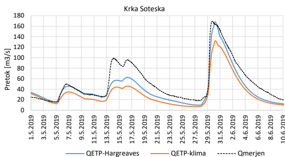
Slika 11: Primerjava simuliranega pretoka z upoštevanjem klimatoloških vrednosti PET in dnevni vrednosti PET z izmerjenimi pretoki na vodomerni postaji Soteska na reki Krki.
