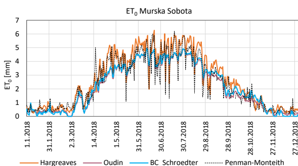
Slika 4: Izsek po različnih metodah izračunanih dnevni vrednosti ET_0 na meteorološki postaji Murska Sobota.
