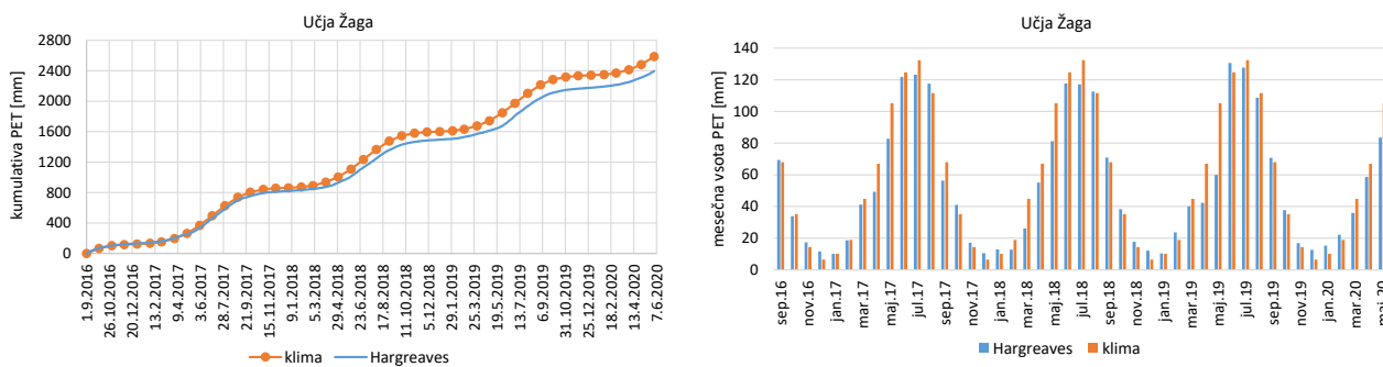
Slika 9: Kumulativna (levo) in mesečna (desno) vsota PET na podporečju Učja Žaga modelskega porečja Soče.
