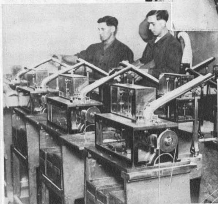
Slika št. 3: Iz prostora, ki ga kaže slika št. 2, pridejo izsekani novci v nov oddelek, kjer jih z avtomatično električno tehniko stehtajo. Novci padajo v tri posode: v prvo dobri, v drugo prelahki in v tretjo pretežki.
