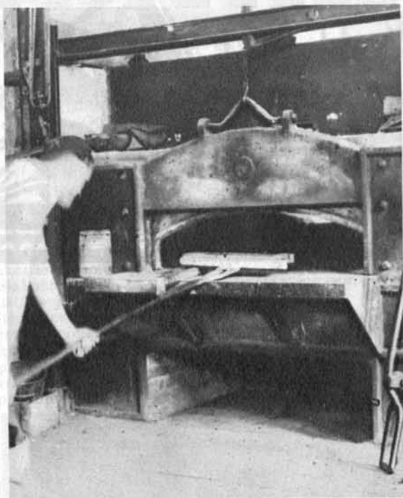
Slika št. 1: V topilnici. Tu se zlate ali srebrne plošče in palice stope in vlijejo iz njih nekaki zlati ali srebrni trakovi v debelini novcev, ki se potem izsekavajo iz trakov.
