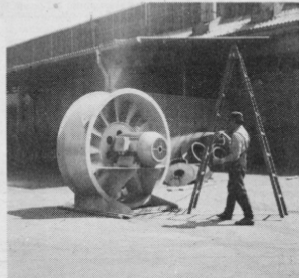
Aksialni ventilator, pretežno namenjen za vgradnjo v industrijske klimatske naprave z velikimi zmogljivostmi. Prav z razvojem tega ventilatorja je stopila Klima v vrsto z najboljšimi proizvajalci v Evropi in v veliki meri zadovoljila do sedaj le uvozne zahteve.
