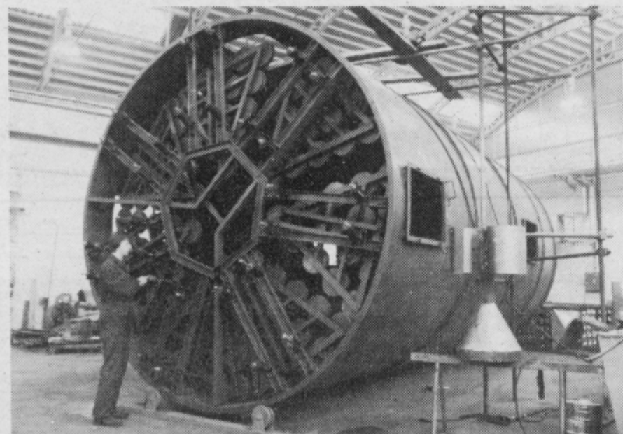
SPF - stolpni platneni filter, pretežno namenjen za filtracijo zraka v lesni industriji, čeprav je primeren tudi za druge industrijske panoge. Je pomemben varčevalec z energijo, kajti filtrirani zrak se vrača v proizvodno dvorano in stroški ogrevanja so manjši.
