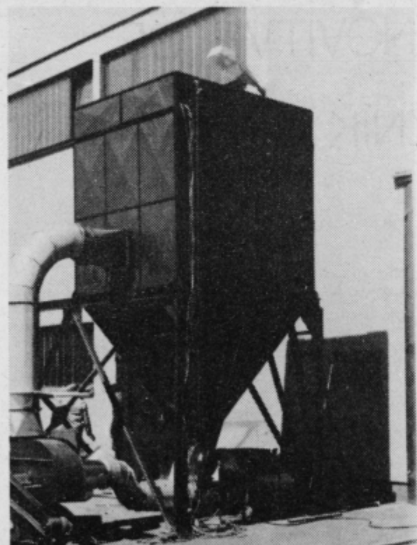
Filter za odpraševanje (prototip) finih prašnih delcev z visokotlačnim zrakom, krmiljen elektropnevmatsko je izdelek in rezultat domačega znanja. Omočga prodor v odpraševanje najbolj zahtevnih materialov in je namenjen uporabi v različnih industrijah.
