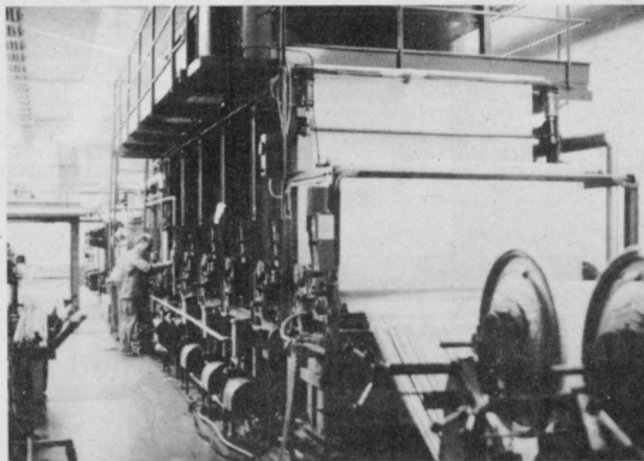
Stroj, ki ga vidimo na obeh slikah so v celoti izdelali v tekstilni tovarni Prebold. To je tako imenovan indigo stroj, ki je popolnoma avtomatski. Deluje na principu nalaganja original indigo barvila na osnovo. Barvilo nanesejo samo na površino preje, tako da vlakno v notranjosti ostane naravne barve. S tem strojem, ki so ga, kot že rečeno, v celoti izdelali doma, so sebi in družbi prihranili precej deviz, kar je v sedanjih gospodarskih prizadevanjih velik plus. Še večji pa je, če vemo, da so stroj izdelali že pred leti, ko so se v Preboldu prav tako kot danes, obnašali stabilizacijsko. Dosežek pa hkrati govori o tem, da so preboldski tekstilci zares veliki strokovnjaki.
