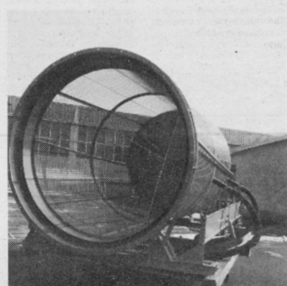
Rotacijski filter za odpraševanje v sistemu klimatizacije v tekstilni industriji. Za te filtre so v Klimi edini proizvajalci v Jugoslaviji. Do sedaj smo jih morali uvažati, zato je Klimin prispevek toliko pomembnejši, saj so rešili problem uvoza te opreme.
