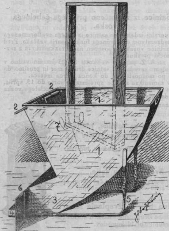
Št. 114. Sipalnik »Ideal« (Stojkovičev) za A. Ž. panj.
