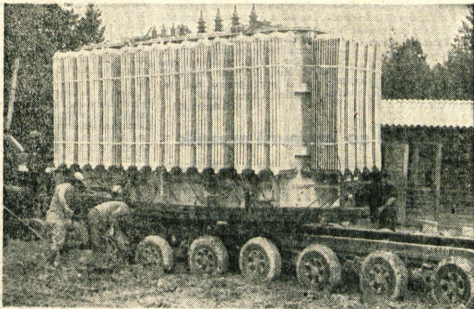
Podjetje Hidromontaža Maribor je pripeljalo v četrtek v Kranj transformator za novo razdelilno transformatorsko postajo na Laborah, ki bo začela obratovati letošnjo jesen. Transformator, ki so ga v četrtek pripeljali v Kranj, tehta 59 ton. (Jk) — Foto: F. Perdan
