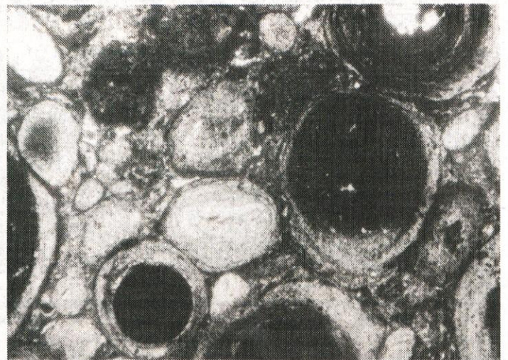
Tako se pod mikroskopom vidi 20 mikrometrov debela boksitna ploščica. Premer največjega zaobljenega zrna je približno 1mm.
