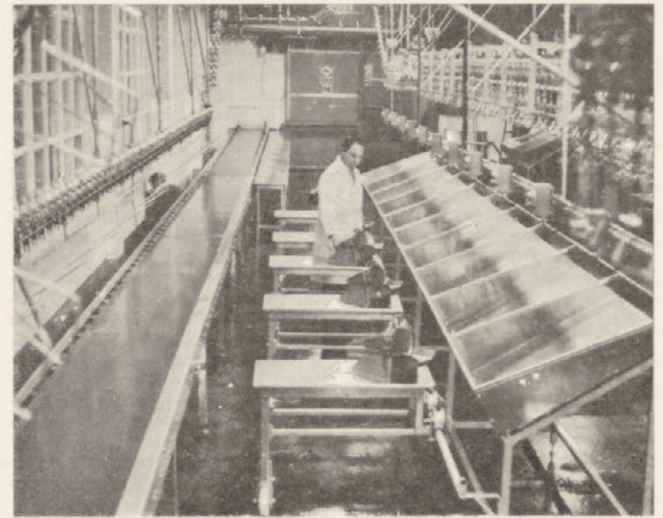
Levo Primatova transportna linija, desno sortirni regali domače proizvodnje
