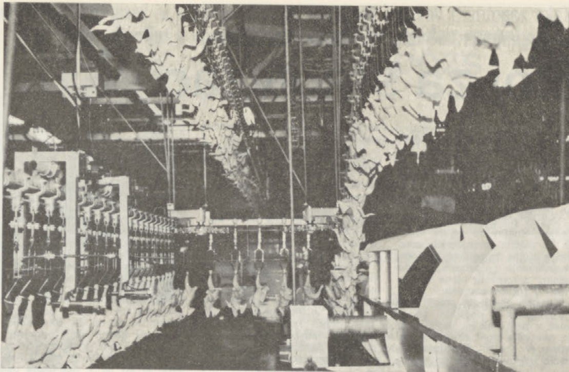
Odcejevalni trak s hladilnim (desno) in sortirnim sistemom (levo)
