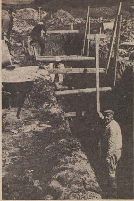
SGP PIONIR nadaljuje jeseni začeto delo na gradbišču Metalne na Senovem. Tovarna gradbenih žerjavov bo na tem mestu stala do jeseni. (Foto: Jožica Teppey)
