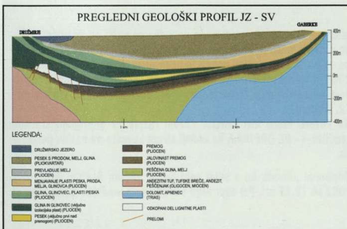
Slika 3: Karakteristični geološki profil
