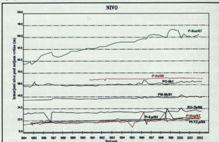
Slika 1: Spremembe nivoja (tlaka) podzemne vode na kvartarnih piezometrih (piezometri segajo do globine cca 200 m)
