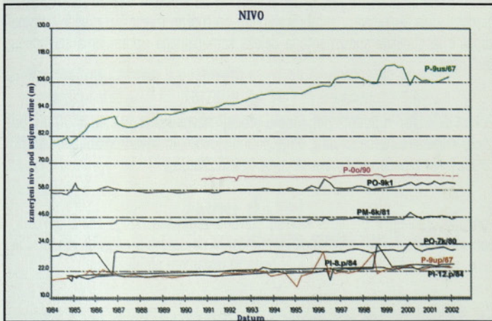
Slika 2: Spremembe nivoja (tlaka) podzemne vode na kvartarnih piezometrih (piezometri segajo do globine nekaj 10 m)
