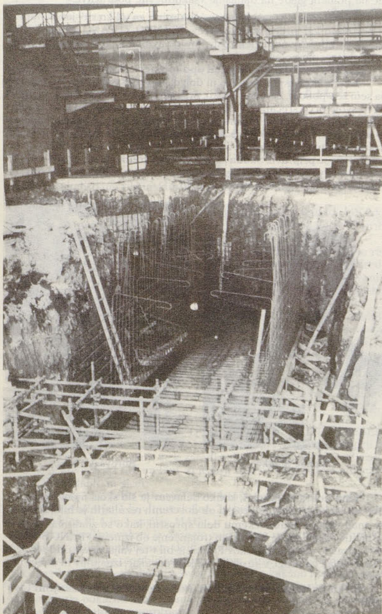
Izvajanje gradbenih del na energetski kineti do strojnice 3 v Valjarni
