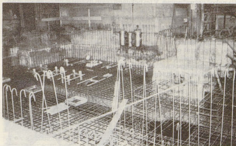
Izvajanje gradbenih del na hidravličnem prostoru strojnice za novo napravo za kontinuirano vlivanje jekla v elektro-jeklarni.
