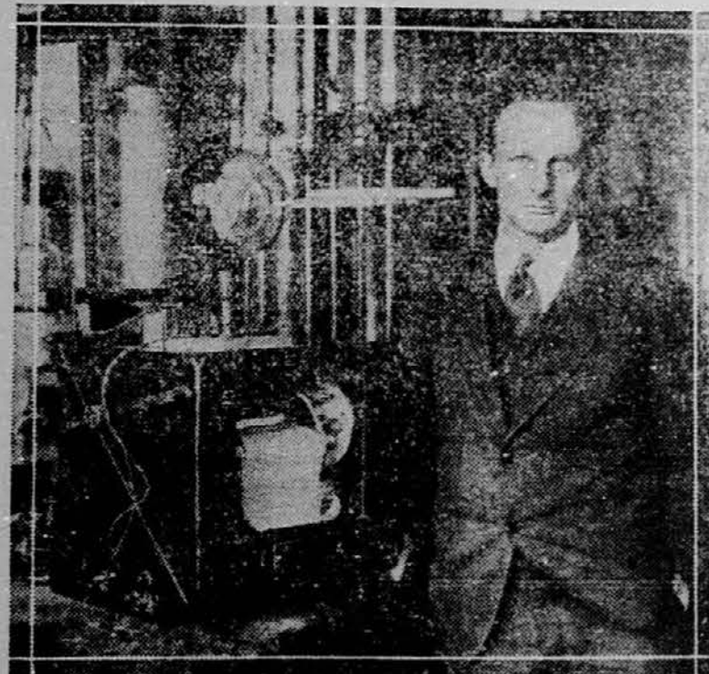
Ko se bo podal to poletje italijanski general Nobile v svojem vodljivem balonu preko Severnega tečaja, bo imel seboj aparat, ki ga vidite na sliki. Z aparatom je mogoče meriti gorkoto polarne luči. Poleg aparata je slika njega iznajditelja dr. L. R. Koller, član General Electric Company.
