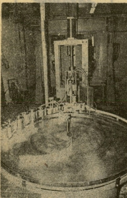
Nova linija: šaržiranje, homogenizacija na vakuumskem planetnem mešalu, avtomatska polnilna linija.
