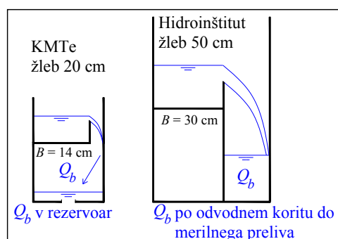
Slika 16: Odvajanje bočnega odtoka Q_b na prelivih v ožjem in širšem koritu
