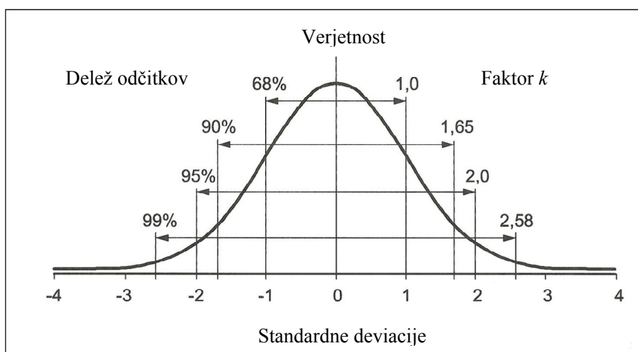
Slika 8: Normalna verjetnostna porazdelitev (ISO 1438:2008, str. 39) Figure 8: The normal probability distribution (ISO 1438:2008, p. 39)
