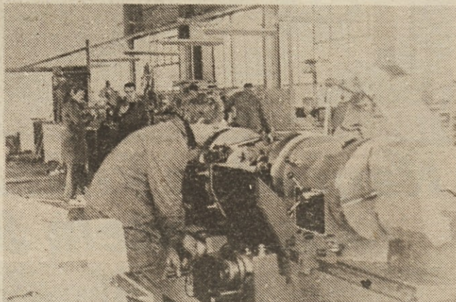
Z novimi stroji, na sliki je specialni stroj za brušenje motornih gredi, opravijo v ptujem Tehnoservis kompletno obnovo motorjev
