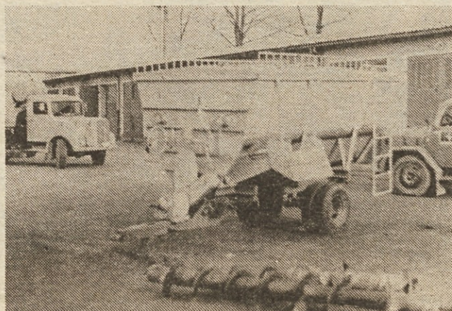
V Tehnoservisu skonstruirana in izdelana prikolica za razvoj suhe krme na živinorejskih farmah je že na voljo kupcem
