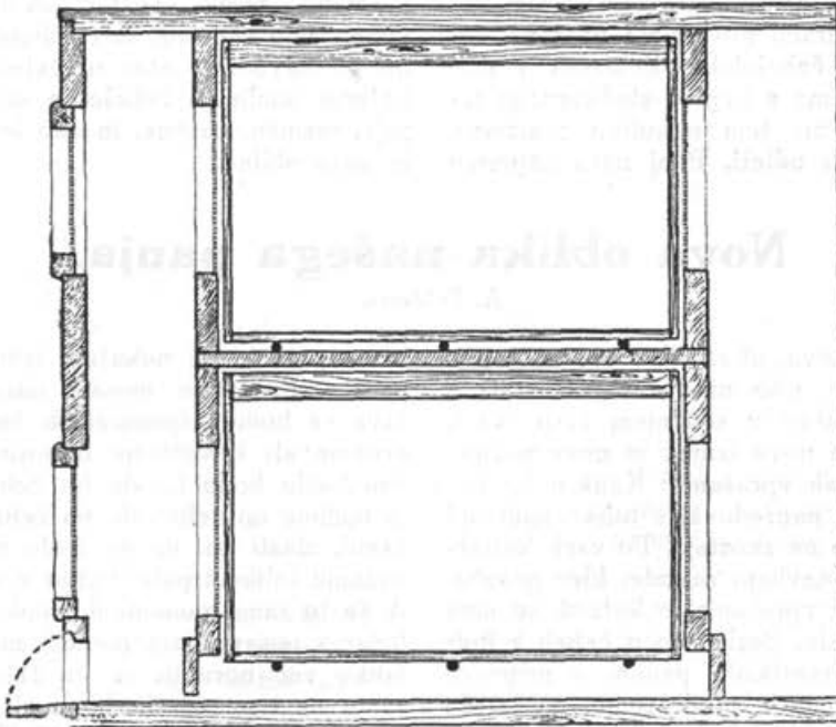
Prerez po dolžini A.-Ž. panja nove oblike.
