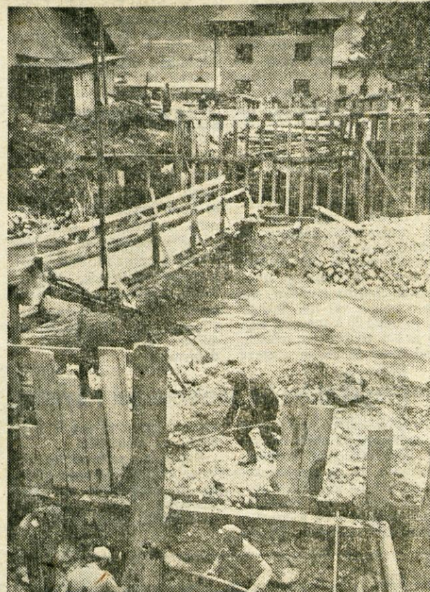
Naselje Podmežaklja na Jesenicah bo, kot obljublja, dobilo že z novim letom dobro zvezo s središčem Jesenic preko mosta, ki je v gradnji. Ta bo širok 11,5 m in 22 m dolg. zgrajen z montažnimi elementi in prednapetim betonom. To bo prva taka gradnja na Gorenjskem. Investitor je jeseniška občina, izvajalec del pa SGP Gradis, s svojo PE na Jesenicah
