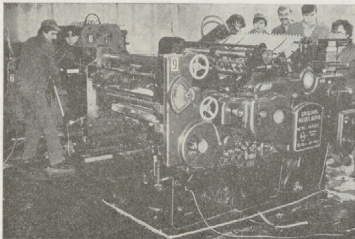
Cilindrski tiskarski stroj HEIDELBERG
