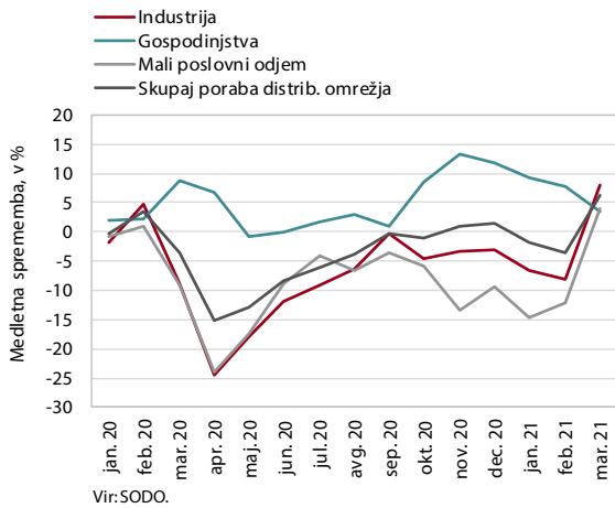
Slika 5: Poraba elektrike po odjemnih skupinah
