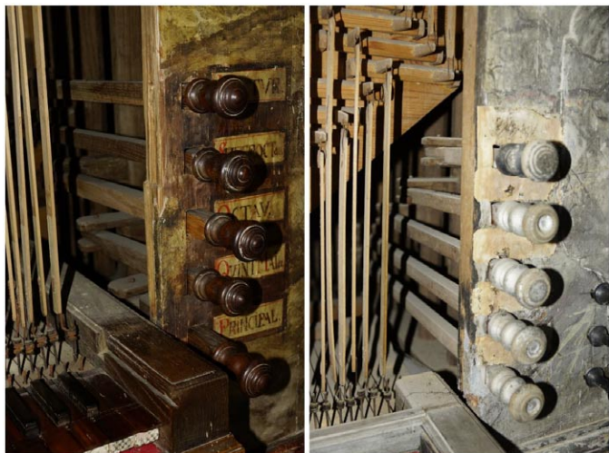
Sl. 9 Podobnost mehanizma v Crngrobu (levo) in Šmihelu (desno).
