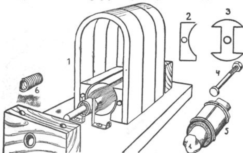
TA SLIKA NAJ VAM POMAGA DA VAM BO LAGLJE ŠLO: 1) slika našega stroja (sprednji ležaj je potegnjen iz osi), 2) pločevina za poljski čevlj, 3) pločevina za kotvo, 4) vijak, ki stiska pločevino poljskih čevljev, 5) kolektor, 6) žični zavoj za strojev ležaj
