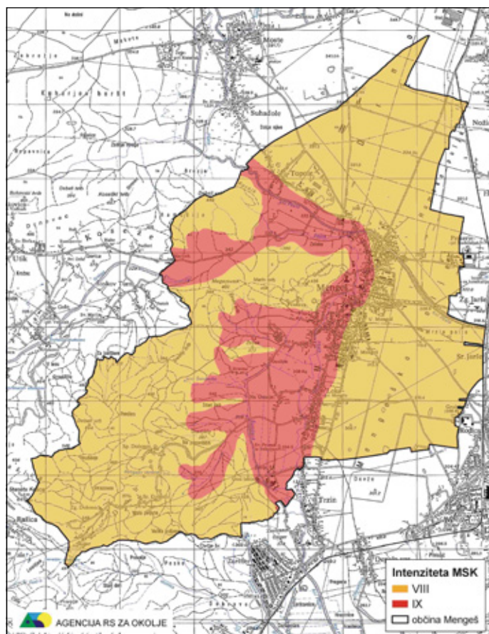
Potresna karta občine Mengeš je verjetno dovolj nazorna, da si lahko predstavljamo njeno nadaljevanje proti jugu na območje sosednjega Trzina. V ravninskih delih občine lahko zato računamo tudi s potresi do IX. stopnje po EMS. (Vir: Urad za seizmologijo in geologijo, ARSO.)
