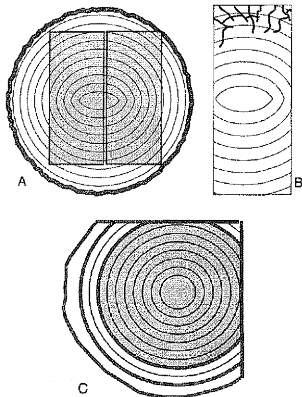
Sl. 3: Trije najpogostejši razlogi za odsotnost terminalne branike: A - tram je ostrorob in je izrezan iz hloda večjega premera, B - periferija trama je preprejena z rovi larv in zaradi tega krhka - pri vrtanju se zato največkrat zdrobi, C - tram je obtesan, beljava in z njo terminalna branika pa odstranjena.
