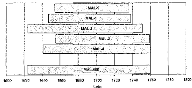
Graf 2: Umestitev povprečnih kronologij za posamezno trikotno vešalo (MAL 1-5) v čas. Na spodnjem delu grafa je prikazana datirana kronologija MAL-900.
