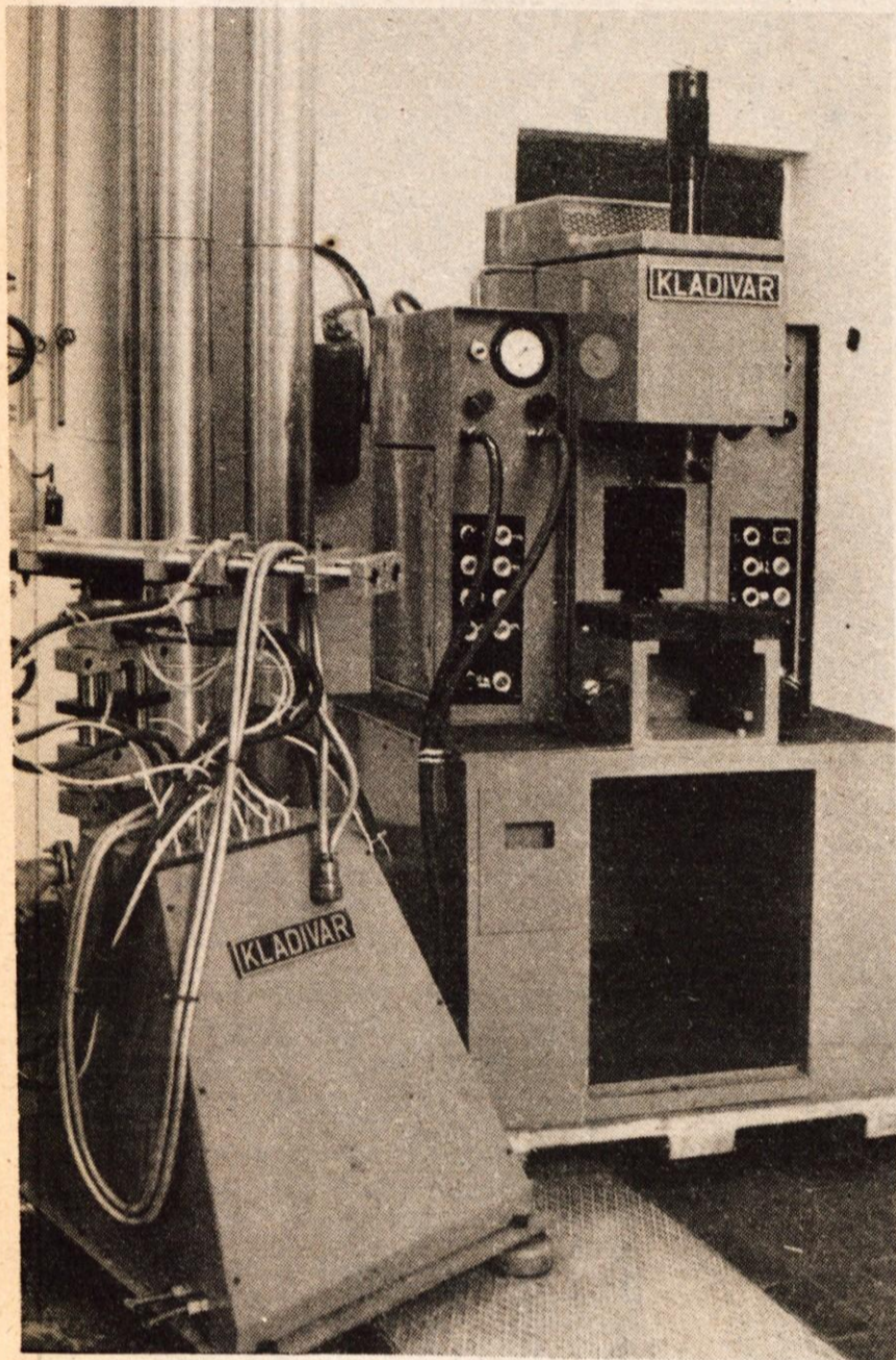
Mehanska roka s področja robotike s hidravličnim preoblikovalnim strojem, ki so ga razvili v Kladivarju.
