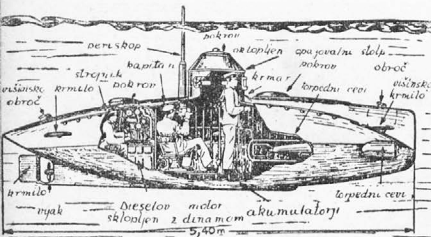
Prerez japonske žepne podmornice s samo tremi možmi. Težka je le okrog 10 ton in nosi s seboj le dva torpeda.
