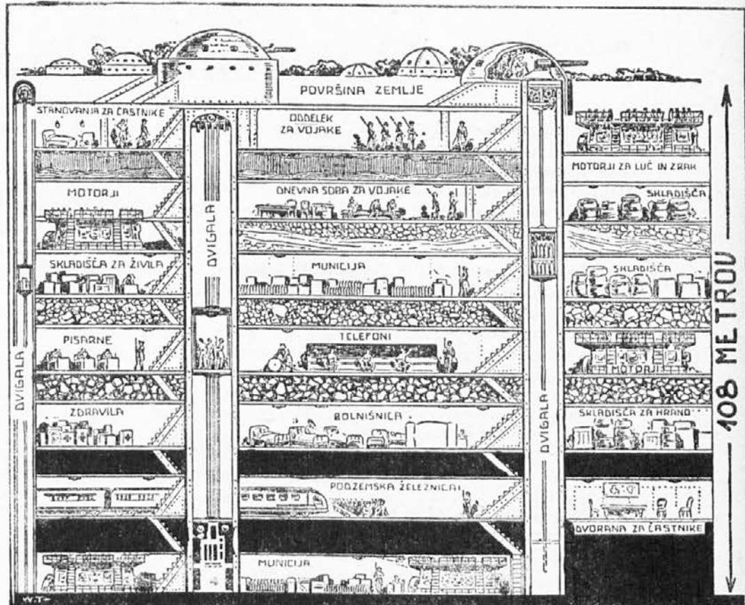
Prerez Maginotove linije.
