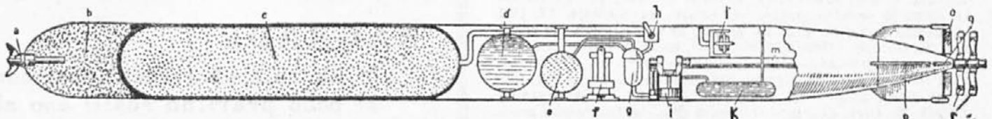
Prerez torpeda: a) vžigač, b) razstrelivo, ki ga je v torpedu 100 do 200 kg, c) kotel za stisnjeni zrak, ki žene motor torpeda; zrak je pod pritiskom 150 do 200 atmosfer, d) kotel z vodo, ki je potrebna pogonskemu motorju, e) kotel za gorivo pogonskega motorja, f) naprava, ki uravnava globinsko krmilo, g) razplinjač, h) ventil za dovod stisnjene zraka, i) pogonski motor, k) olje za mažo motorja, l) naprava, ki vodi torpedo ves čas v isti smeri, m) dvojno vreteno, na katerem sta pogonska vijaka, n) stransko krmilo, ki je v zvezi z l), p) globinska plavut, q) globinsko krmilo, r) pogonska vijaka.
