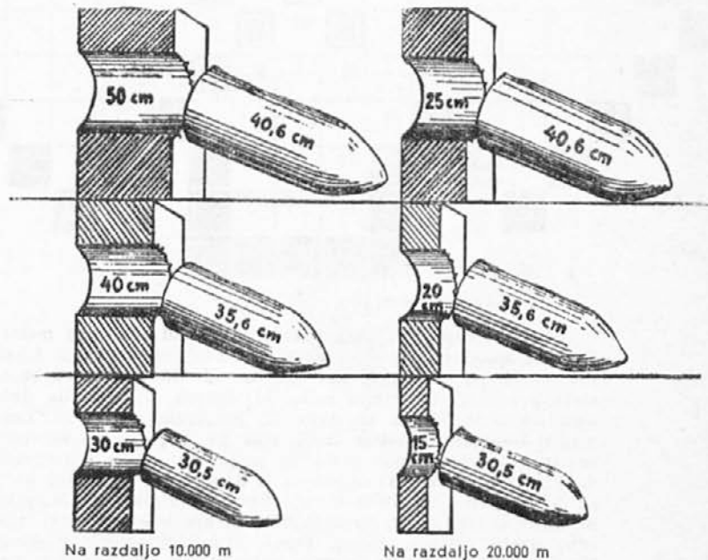
Probojnost granat, ki jih streljajo ladijski topovi. Probojnost je računana na jeklene oklepe glede na kaliber topov in na oddaljenost cilja.
