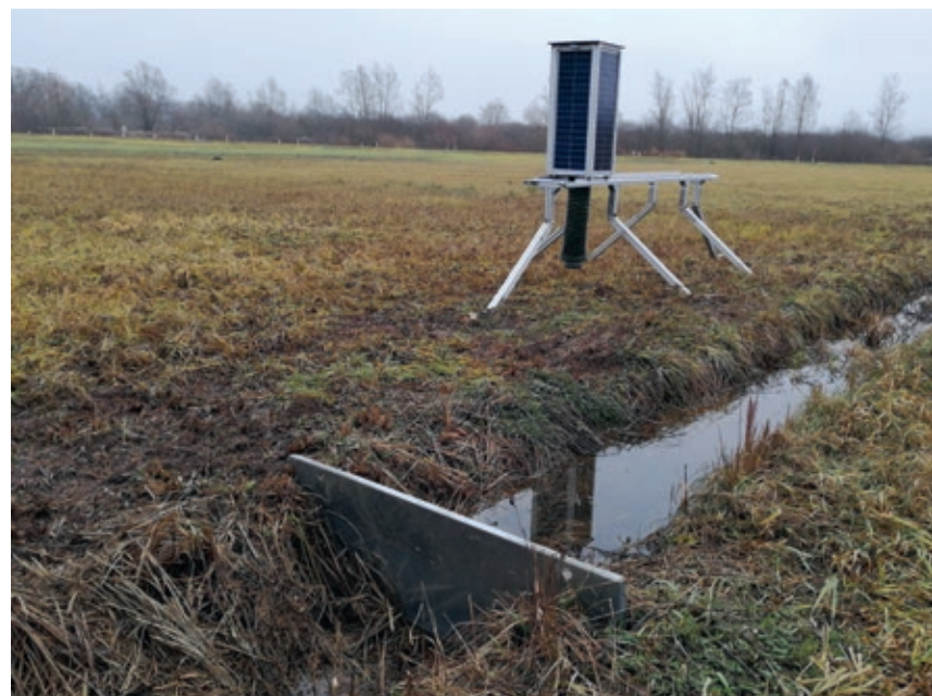
Naprava za merjenje emisij toplogrednih plinov
