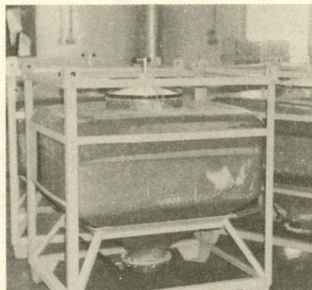
Zalogovniki za pozitivno in negativno maso za proizvodnjo alkalnih baterij
