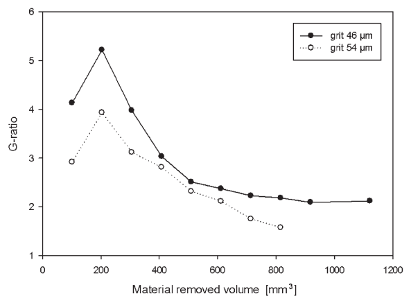
Fig. 8. G-ratio
