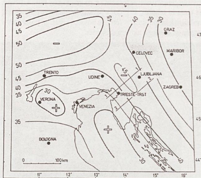
2. Globina Mohorovičićeve diskontinuitete. Po tržaškem geologu G. Carulliju in sodelavcih iz leta 1990.
