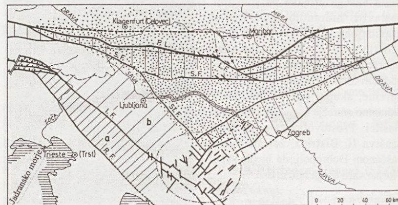
1. S črnimi črtami so vrisani pomembnejši prelomi v Sloveniji. R.F. = Raški prelom, I.F. je Idriški prelom. Skico je izdelal geolog L. Placer leta 1999.
