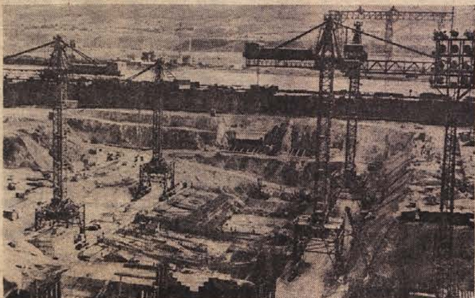
NAJVEČJE GRADBISČE V EVROPI. Takšno podoba kaže te dni gradbišče djerdapske hidrocentrale, kjer bo zajezena Donava dajala čez nekaj let okoli 11 milijard kilovatnih ur električne energije — skoraj toliko, kot jo zdaj na leto porabi vsa Jugoslavija! Del opreme je za to hidrocentrale prispevala tudi krmeljska Metalna. Zgornji posnetek je z romunske strani. (Foto: Marjan Legan)
