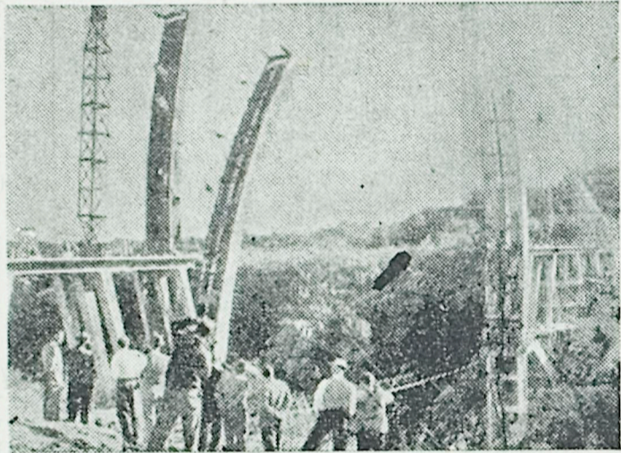
Čez reko Storms v Južni Afriki so zgradili skoraj 200 metrov dolg jekleni most, ki se boči nad 125 metrov globoko sotesko. Obe, več deset ton težki »rebrici« so sestavili na bregu, nato pa so ju z dvigali počasi spuščali drugo proti drugi, da sta se sredi soteske ujeli. To je bil prvi poskus gradnje tako velikega mostu na ta način, kar pa je popolnoma uspelo.
