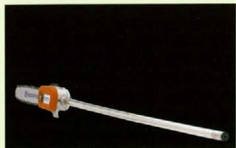
Višinski obrezovalnik Husqvarna z deljivo cevjo za lažje shranjevanje in prenašanje z dosegom do 5 m
