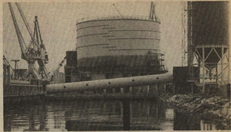
Silos za glinico v Luki Koper stoji na temeljih, ki so jih naredili de-lavci tozda GE Koper. Kompletan objekt stoji na pilotih.
