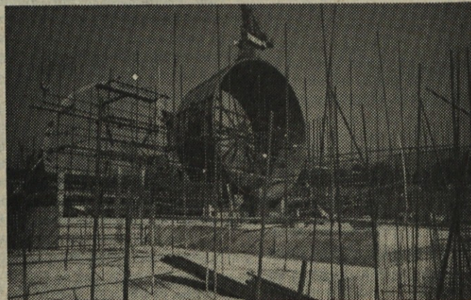
Priprava na betoniranje turbinskega jaška v HE Vrhovo.
