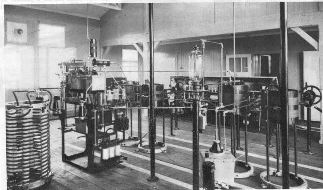
Oddajna aparatura naše radio oddajne postaje v Domžalah, ki se je zadnje mesece jako izpopolnila.
