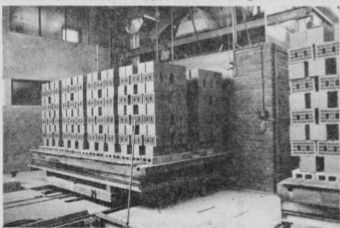
Opeko žgejo v sodobni tunelski peči.
