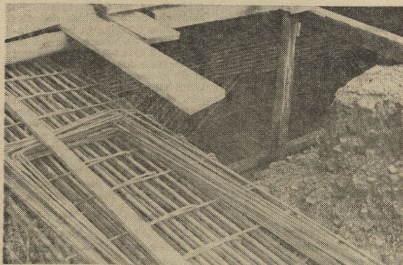
Jeklene armature temeljnega nosilca
