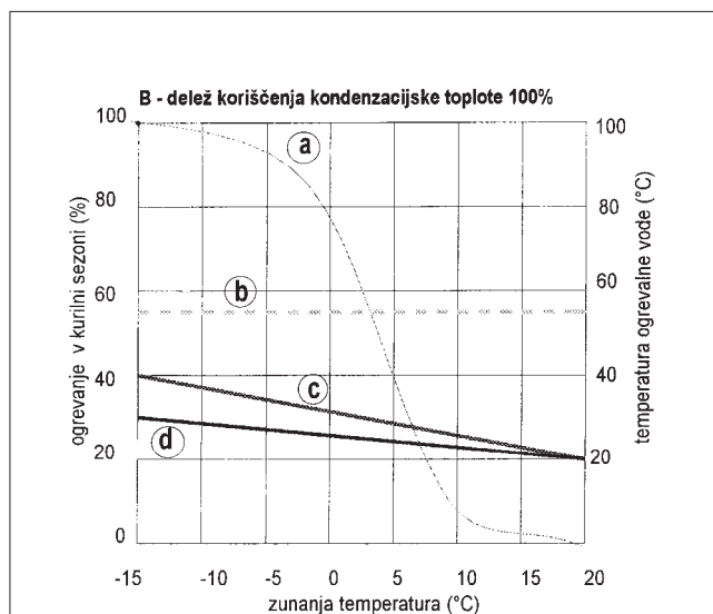
a .. krivulja ogrevanja v kurilni sezoni b.. meja kondenzacije za zemeljski plin c.. pretok d.. povratek
