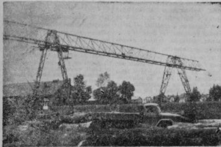
50-tonski žerjav v žagarskem obratu v Rogoznici
