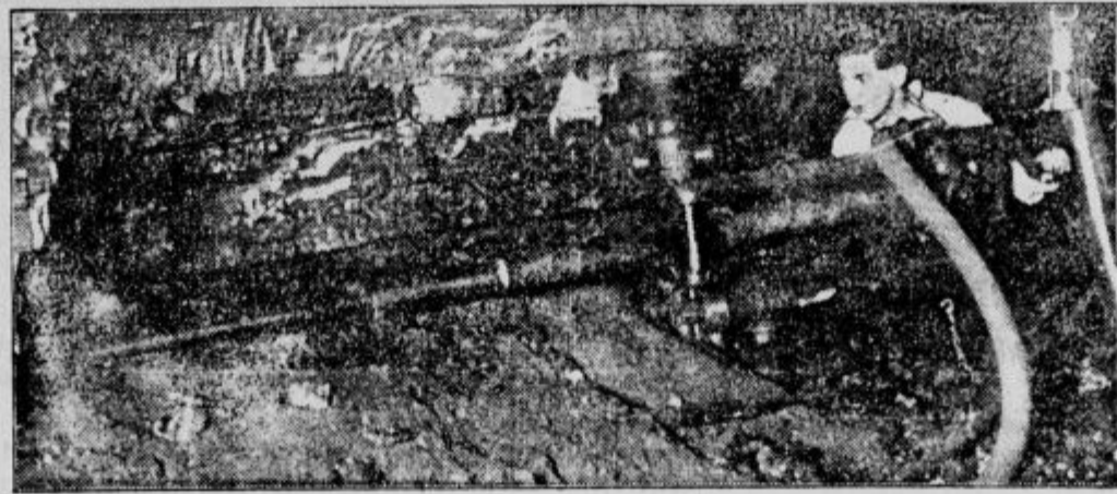
Delavec koplje s vrtnalnim strojem na stianjeni srak luknjo, v katero vliči mino.
