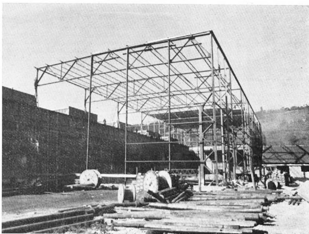
Montaža težke mehanske obdelovalnice
