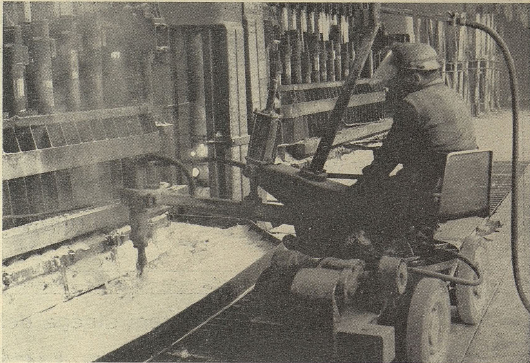
Prebijanje skorje
