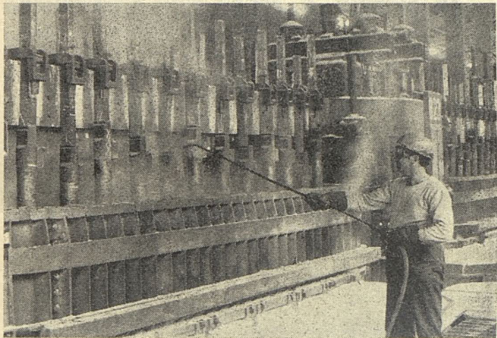
Izpihavanje anod
