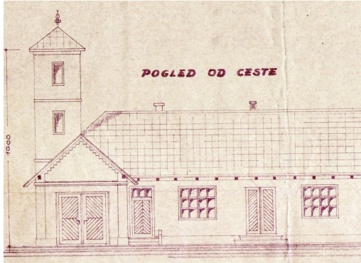
Detajl načrta gradnje dvorane in stolpa v Radomerju
