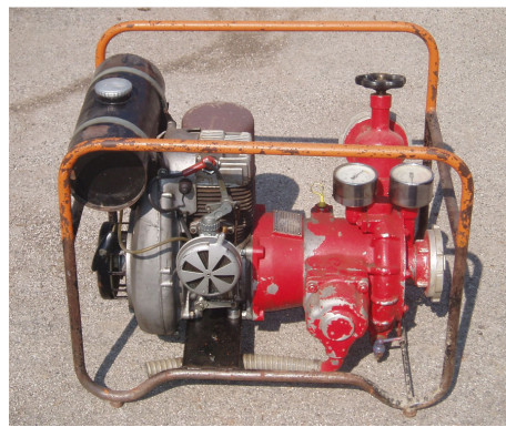
Motorna brizgalna »Ziegler 5/5«
