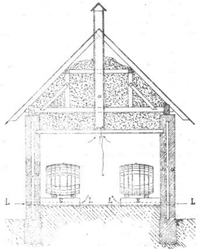
Podoba št. 1. Poprečni presek nadzemljske vinske kleti.
