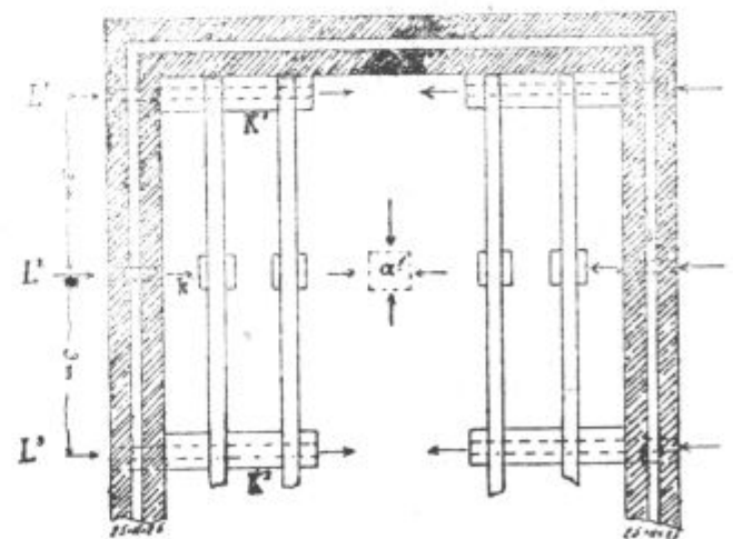
Podoba št. 2. Tloris nadzemljske vinske kleti.
