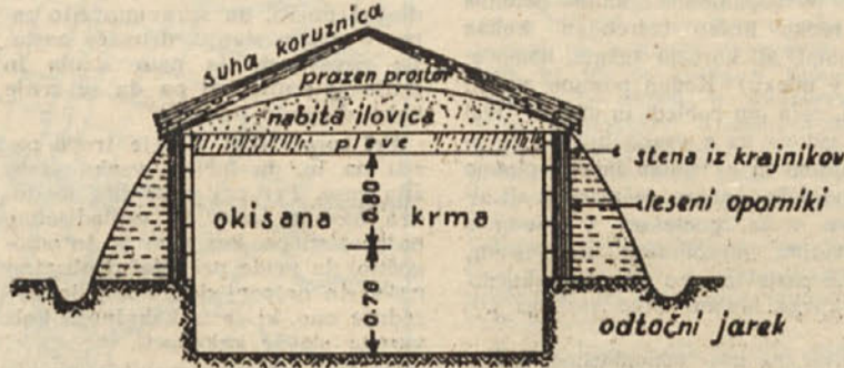
Prikaz preproste jame za kisanje krme
