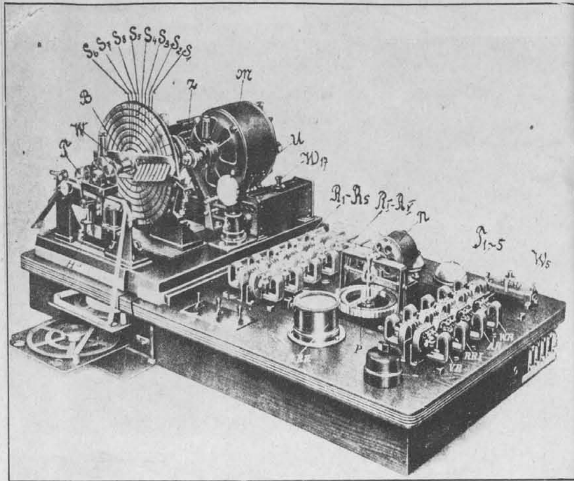
Avtomatičen strojni brzojav. (Glej članek v današnjem »Slovenec«.)
