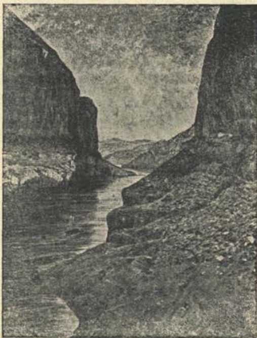
Velika kitajska reka Jangcekjang si je na svoji poti proti morju izjedla okrog osem sto kilometrov dolg prekop, imenovan »Rdeče korito«, skozi diluvialne plasti zemlje.
