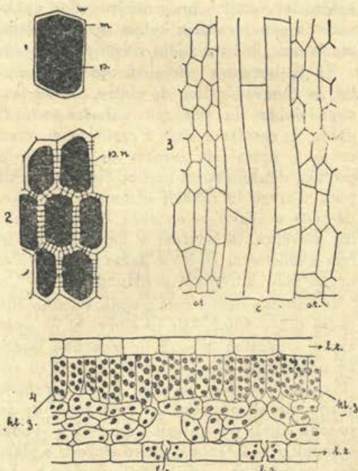
1. Celica: m = mrenica, p = plazma. — 2. Celice v mahovem listu: pn = plazmatične niti. — 3. Podolžni prerez skozi stebelce: c = cevi, st = celice. — 4. Prečni prerez skozi list: lt = listna tančica, ali kožica, lr = listna reža, klz = klorofilova zrnca.
