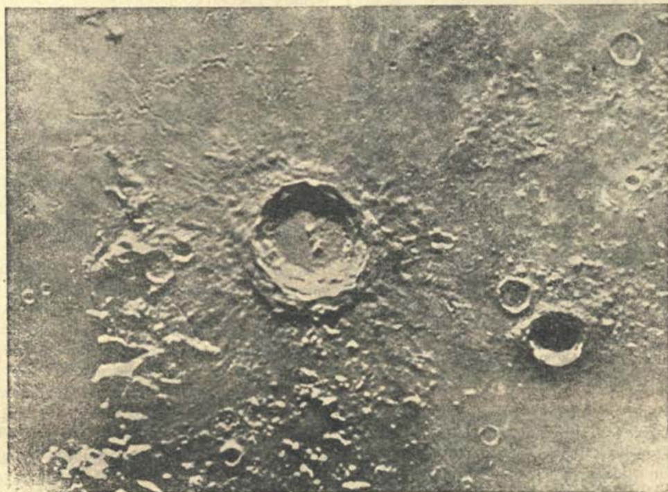
Krožno pógorje Kopernik in okolica na luni (fotografirano v amerškem observatoriju Yerkesu).
