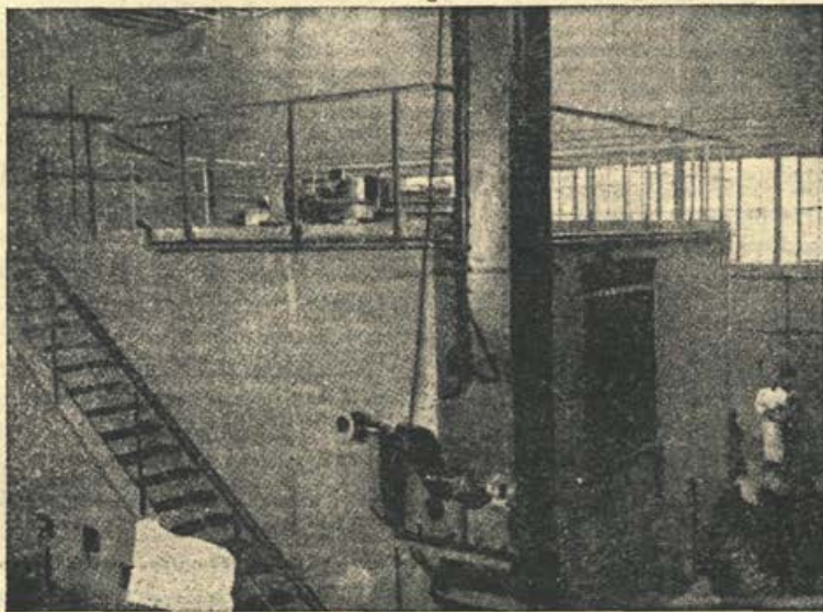
Pogled na uranski kotel, ki so ga postavili Francozi v Chatillonu. Delati je začel decembra 1948.
