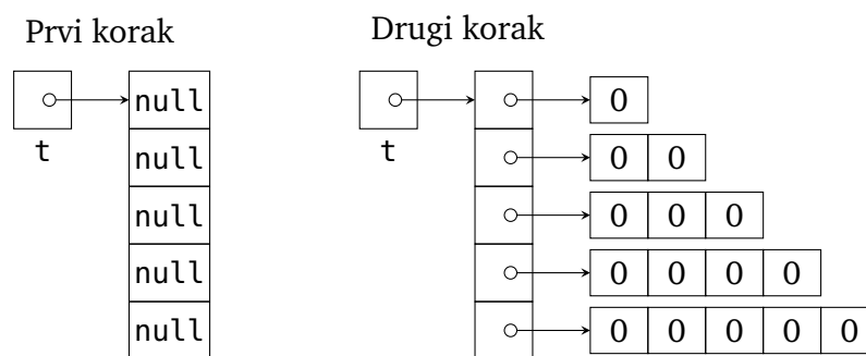
Slika 5.14 Dvostopenjska izdelava dvodimenzionalne tabele.
