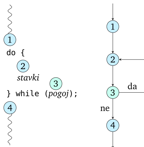
Slika 3.4 Izvajanje zanke do .
