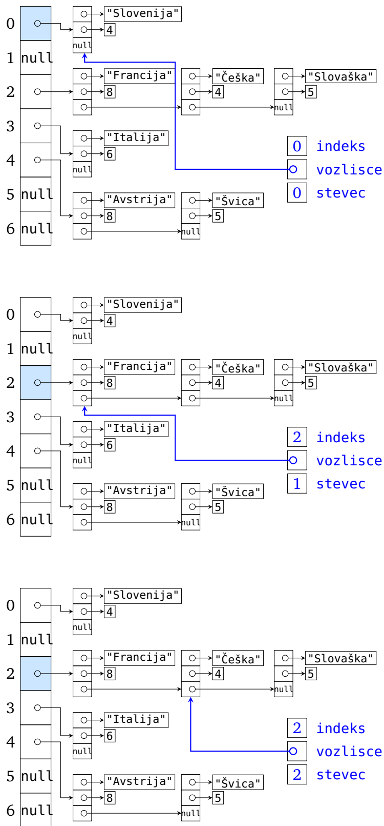
Slika 9.1 Prvi trije koraki sprehoda iteratorja po zgoščeni tabeli.
