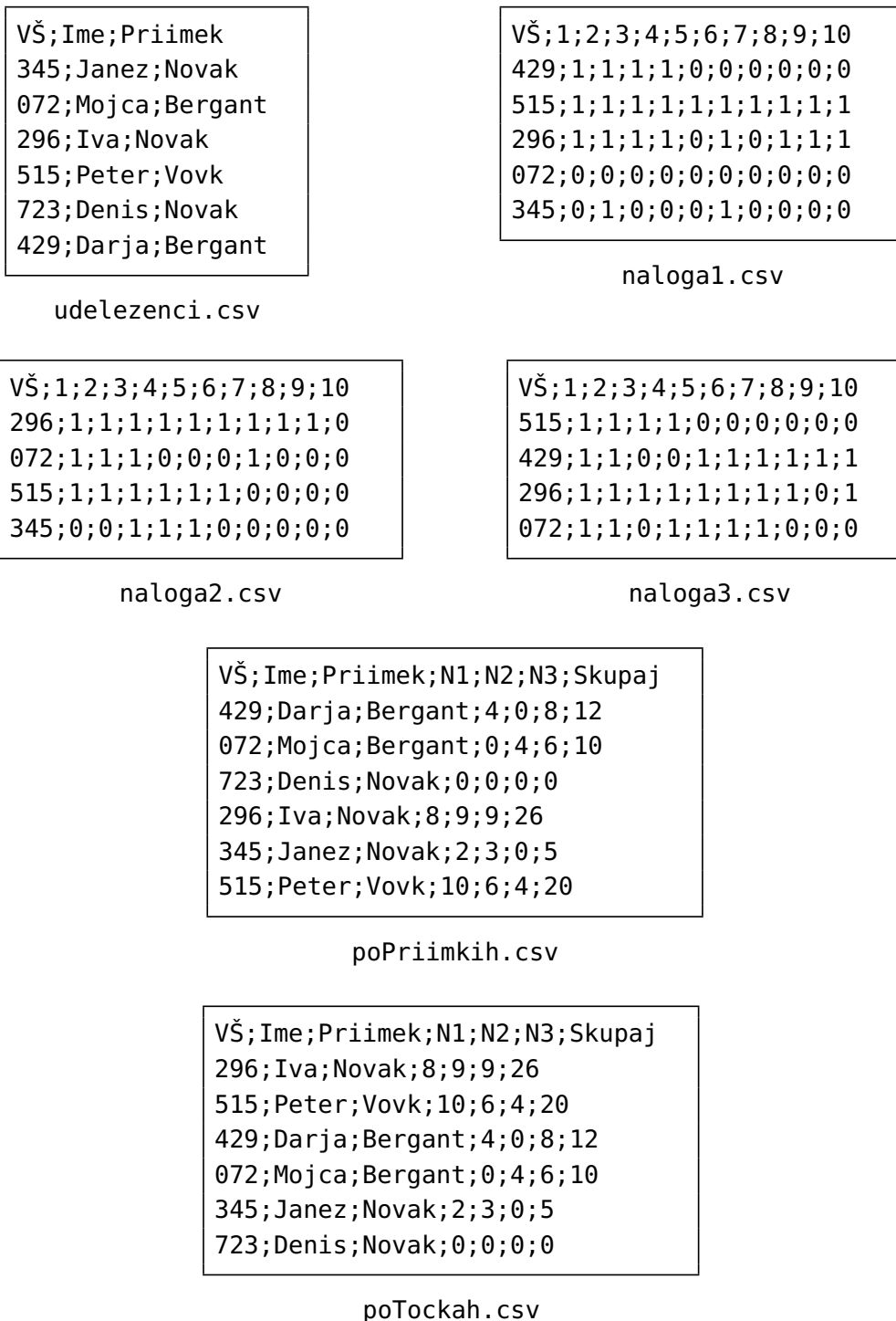
Slika 11.1 Program za obdelavo rezultatov izpita na podlagi datotek udelezenci.csv, naloga1.csv, naloga2.csv in naloga3.csv izdelava datoteki poPriimkih.csv in poTockah.csv. V arhivu ZIP na spletni strani knjige so datoteke dostopne v imeniku lambde/obdelavaRezultatovIzpita.
