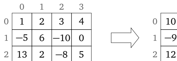
Slika 5.15 Vsote posameznih vrstic dvodimenzionalne tabele.
