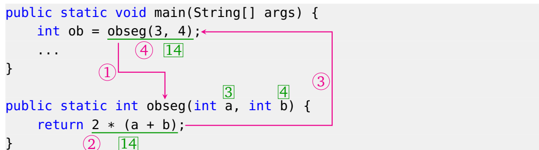
Slika 4.2 Klic metode, ki vrne vrednost.
