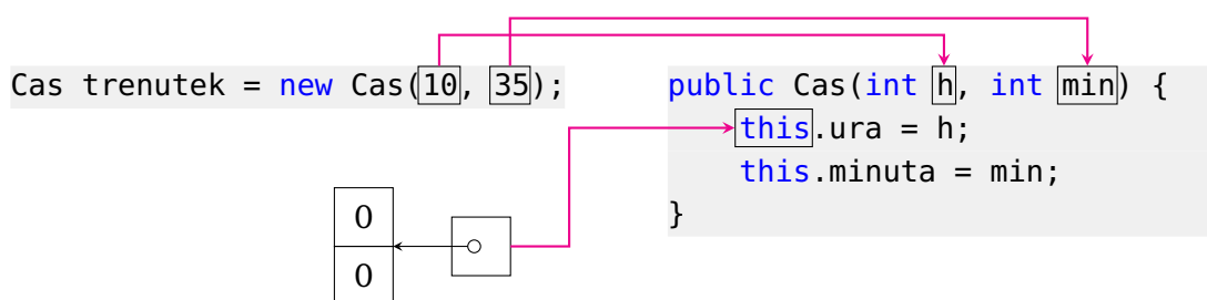
Slika 6.4 Klic konstruktorja.
